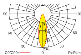
Lampenlichtstrom: 280 lm
